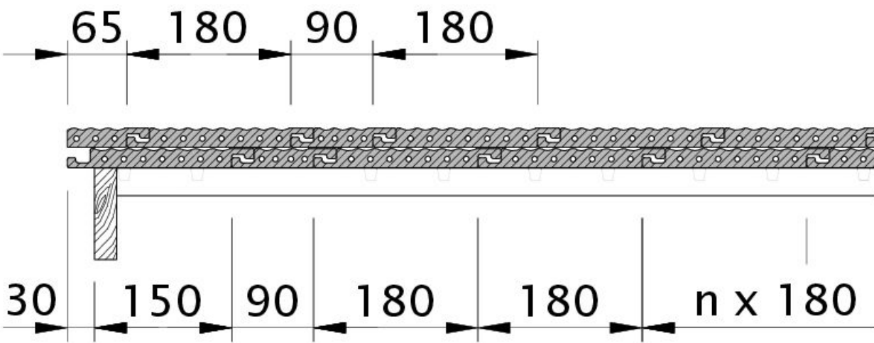
Zeichnung PROFIL Ortgangziegel rechts mit Ortgangbrett OBR
