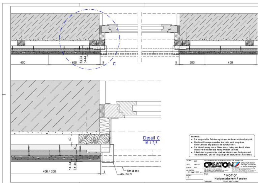
Zeichnung MOTIO Horizontalschnitt-Fenster
