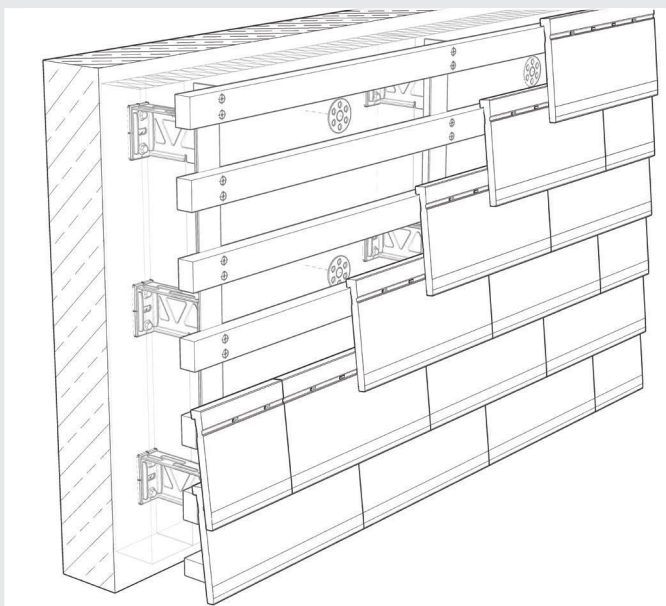
Veranschaulichung Alu/Holz
