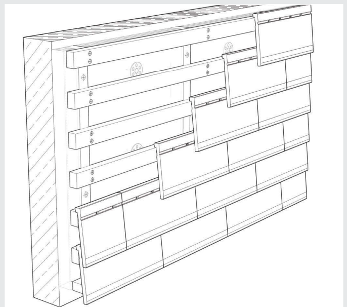
Veranschaulichung Holz/Holz
