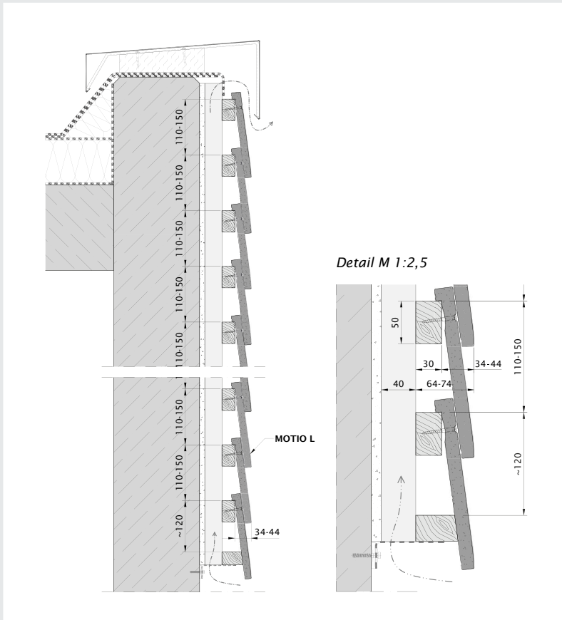
Vertikalschnitt
